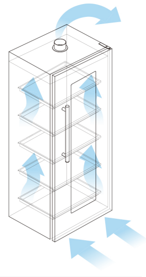
유체 흐름도
